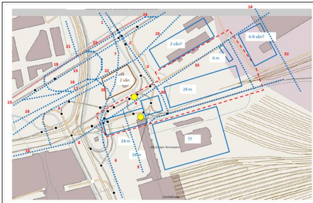
Figur 13: Översiktlig bild över Centralstationsområdet i alternativ med Västlänken. Ljusblå block symboliserar nya hus. Gula cirklar är frånluftstorn. Ljusblå punktlinjer markerar nya vägar. Röda siffror markerar ut gator där trafikmängder kommer att förändras i samband med Västlänken.
